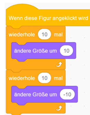
7 Der Buchstabe wird beim Anklicken größer und kleiner.
